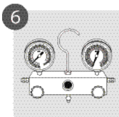
6 Вакумируйте систему охлаждения
